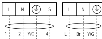
Внутренние блоки
